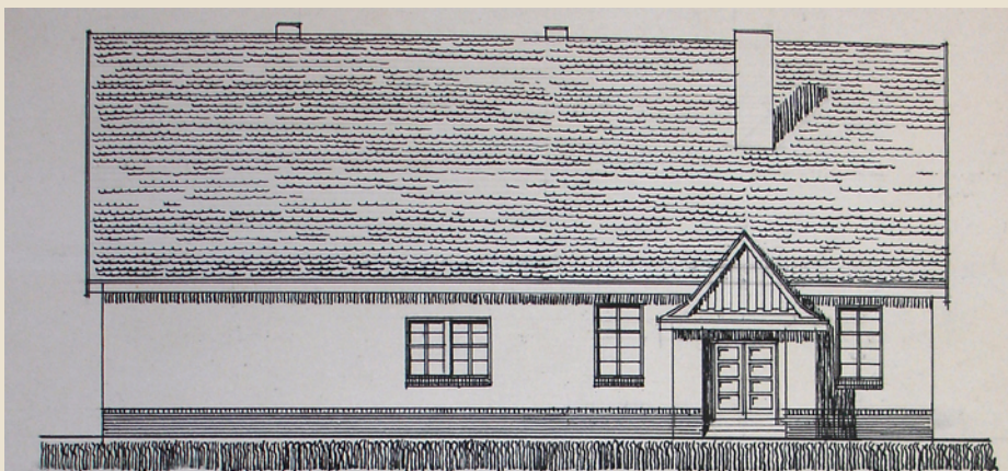
Szkic elewacji szkoły w Żydowie (dokumentacja budowlana), 1911 r., Archiwum Państwowe w Poznaniu
